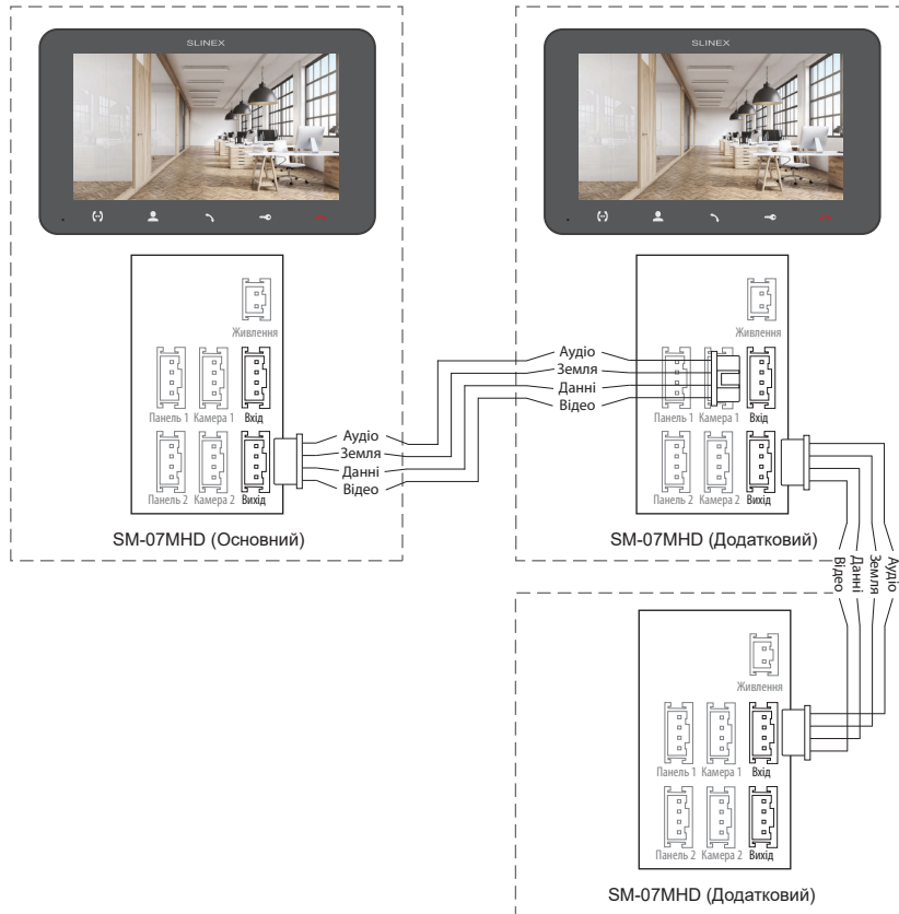
Схема 2. Підключення системи домофонів SM-07MHD
